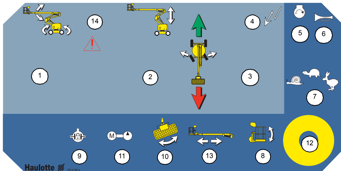
Foto 4: Pupitre de mando «barquilla»
