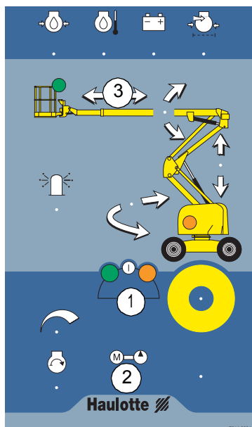
Foto 9: Mando de emergencia
