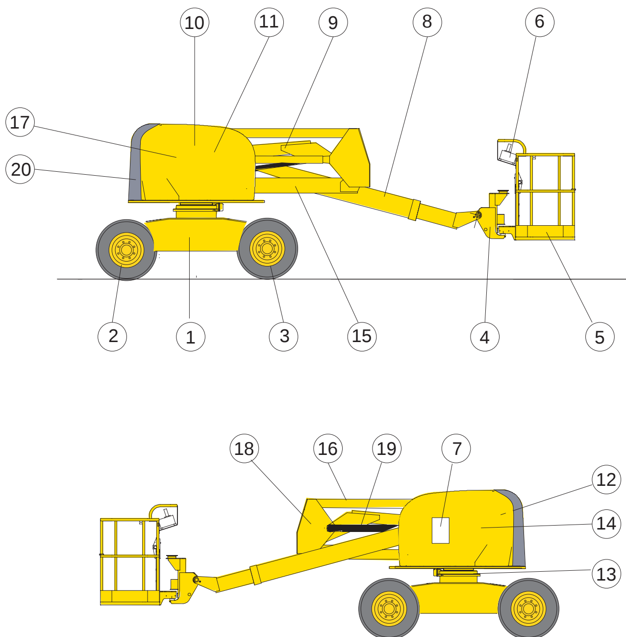
Fig. 2 - Principales Componentes
